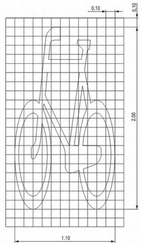
Rys. 5.2.9.1. Znak P-23
